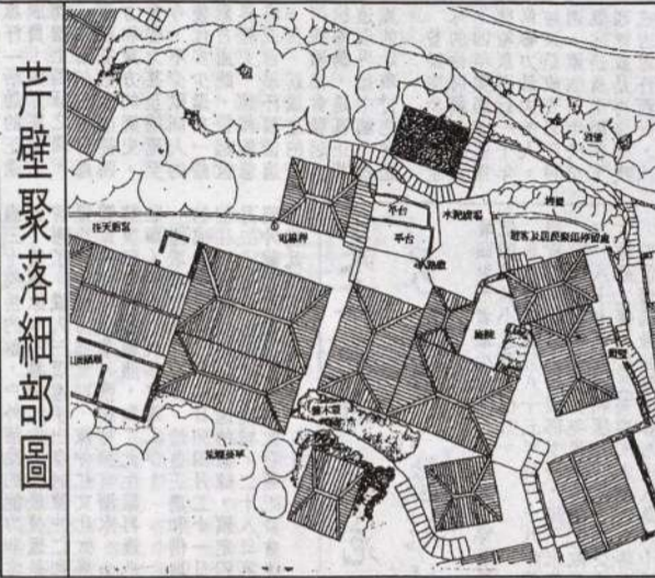
芹壁聚落細部圖
