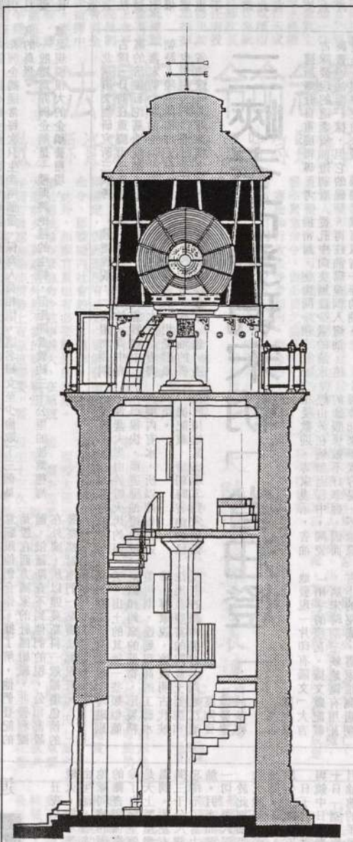
東犬燈塔剖面圖
