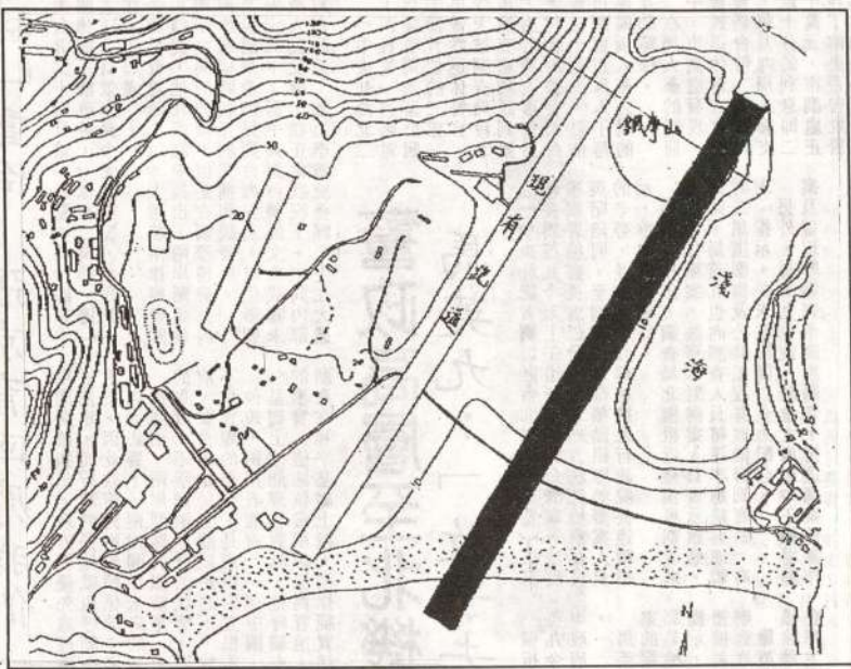
圖一：北竿機場第二跑道位置圖。圖中紅色線段為第二跑道位置，黑色線段為第一跑道位置。
