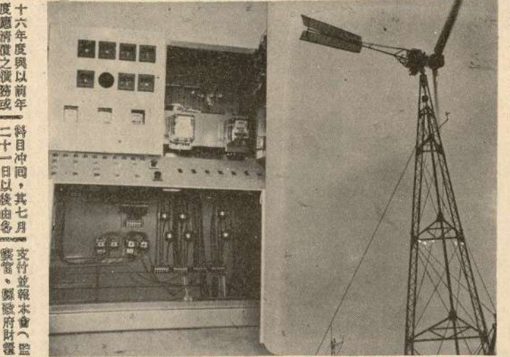
風力發電設備，圖為電力控制機，右為一般家庭用品四瓦風機。(宋志富攝)
