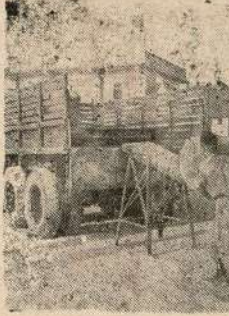
港勤部隊研製的簡易裝車架(嚴正攝)
